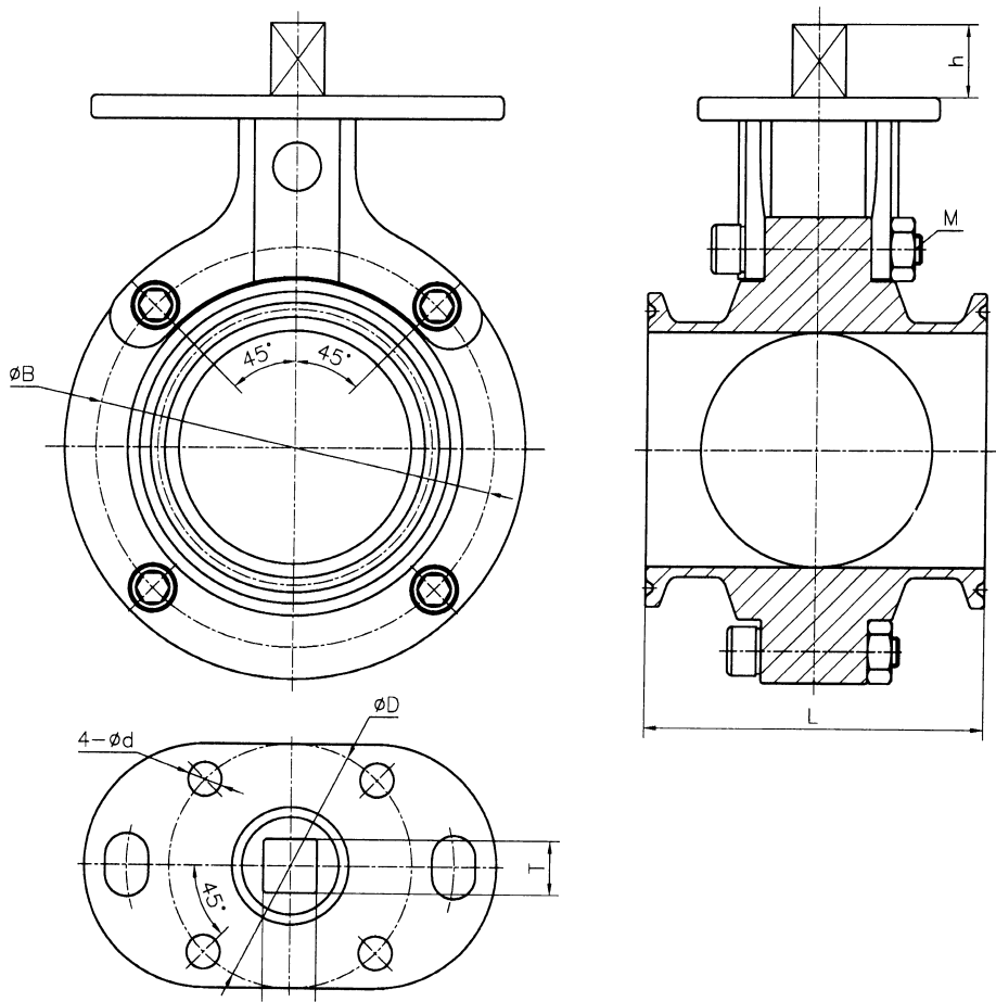
FRONT · SECTION · PLATFORM VIEW · DIMENSIONS PER TABLE · UNIT: MM
