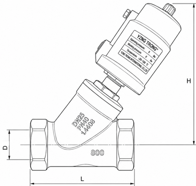
ASSEMBLY DRAWING · UNIT : MM · MATERIAL : CF8M (SS316)
